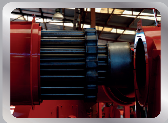
Топочный блок
